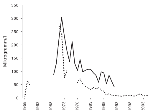
Abb. 5. Entwicklung des Phosphorgehalts 1958–2005 (unvollständige Messreihen). Ausgezogene Linie: Gesamtphosphorgehalt im Stausee Niederried; punktierte Linie: Ortho-Phosphatgehalt bei Hagneck (8 km unterhalb des Niederried-Wehrs). Quelle: Amt für Gewässerschutz und Abfallwirtschaft des Kantons Bern. – Phosphorus content 1958–2005 (incomplete samples). Solid line: total phosphorus content at the Niederried reservoir; dotted line: Ortho-phosphate content at Hagneck (8 km downstream of the reservoir).
